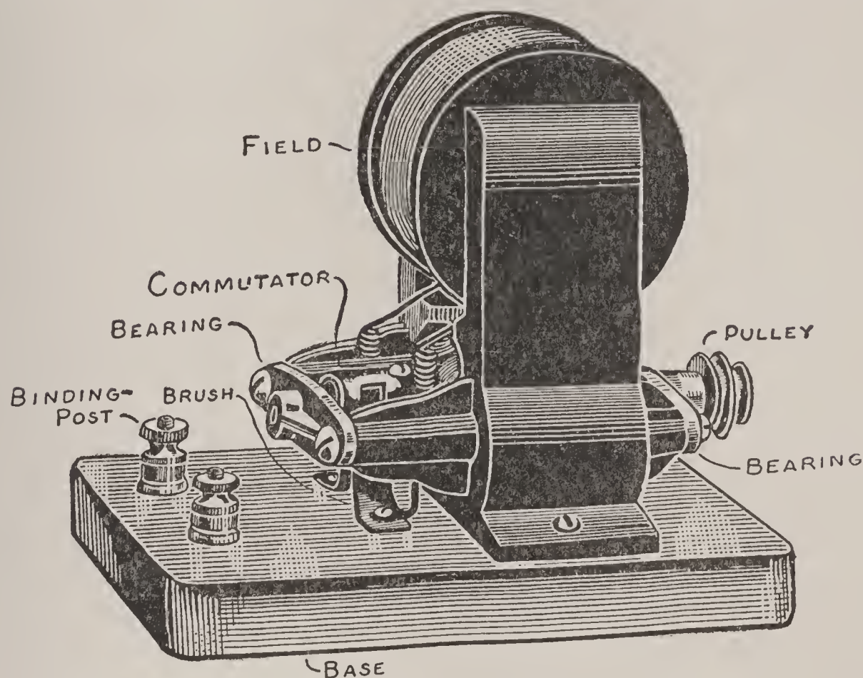
FIG. 267. — Complete Dynamo.
