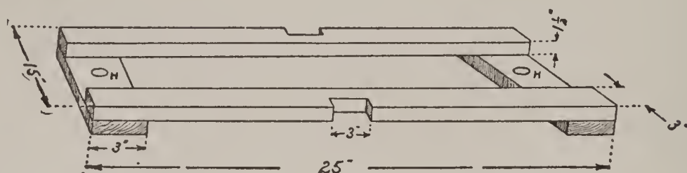
FIG. 37. — The Frame.
