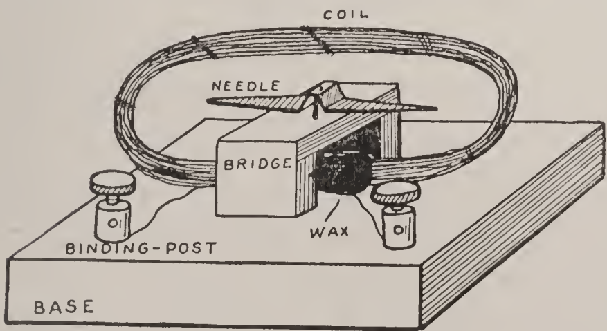
FIG. 111. — Galvanoscope.
