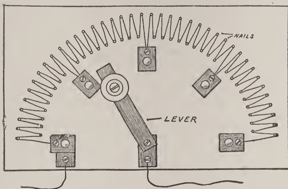
FIG. 318. — A Rheostat.
