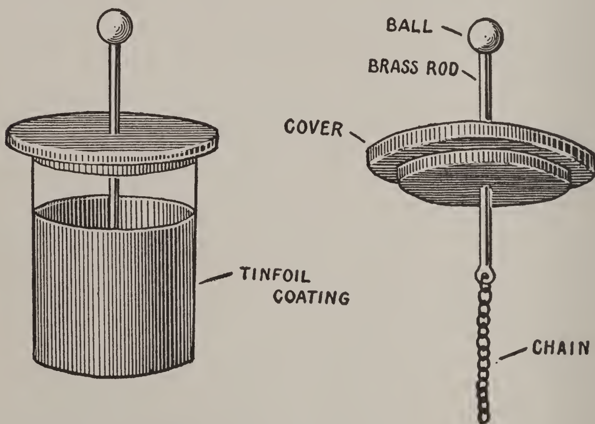
FIG. 45. — The Leyden Jar.
